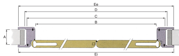
Rever a doppio battente, sezione orizzontale - Two leaves REVER, horizontal section
