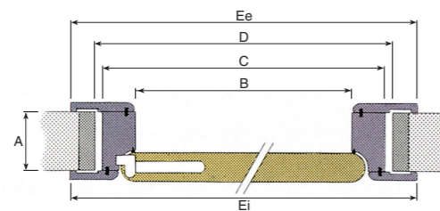
REVER a un battente, sezione orizzontale - One leaf REVER, horizontal section
