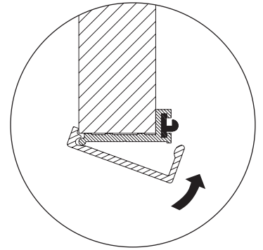
Montaggio su parete in cartongesso Assembling on plasterboard wall
