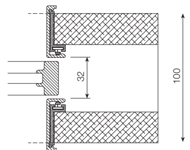
Montaggio su parete in cartongesso Assembling on plasterboard wall
