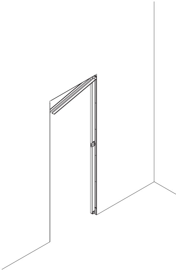
Montaggio su parete in muratura Assembling on brick wall
