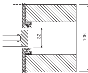
Montaggio su parete in muratura Assembling on brick wall
