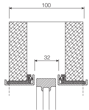
Montaggio su parete in cartongesso Assembling on plasterboard wall
