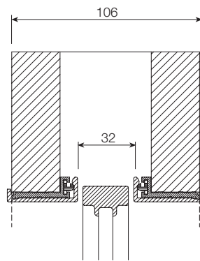
Montaggio su parete in muratura Assembling on brick wall
